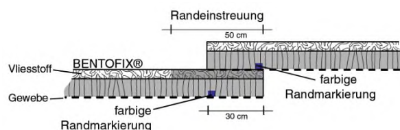
Abb. 4: Schematischer Längsüberlappungsbereich bei einer Kanteneinstreung
