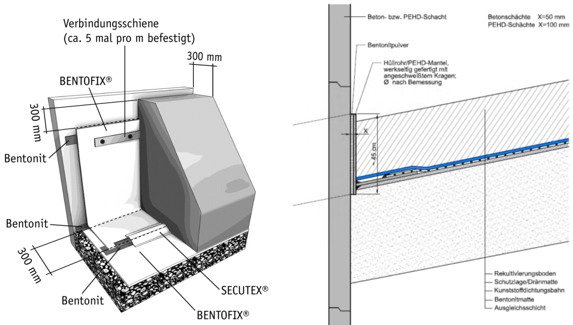
Abb. 12: Bauwerksanschlüsse
