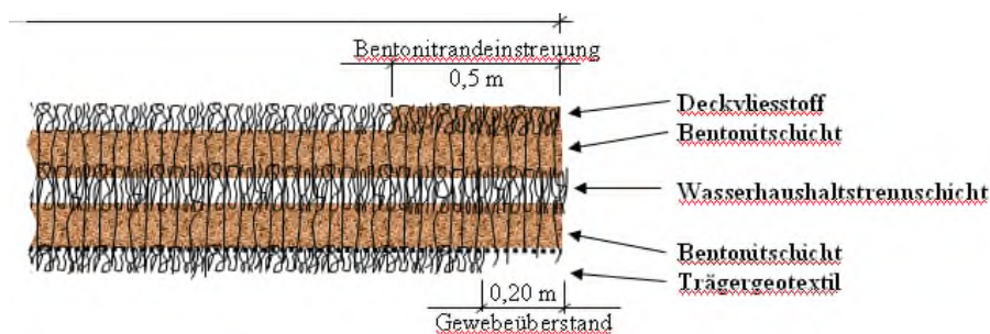
Abb. 1: Schematischer Querschnitt von Bentofix BZ 6000
