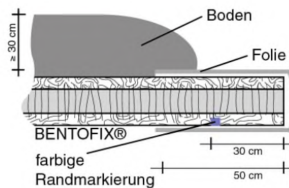
Abb. 14: Baufolienabdeckung
